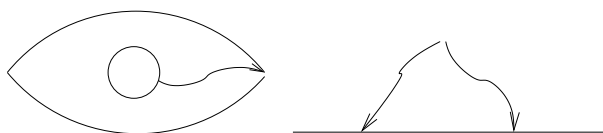
FIGURE 4. Chemin de l'iris jusqu'au coin
