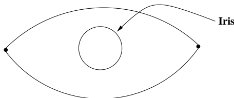
FIGURE 1. La variété \overline{C}_{2,0} .
