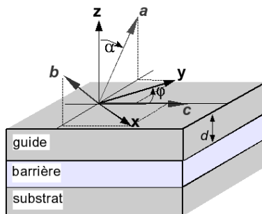
Fig. 1 : Schéma de l'échantillon étudié. a , b , c représentent les axes cristallins et x , y et z les coordonnées du guidage. y est la direction de propagation
