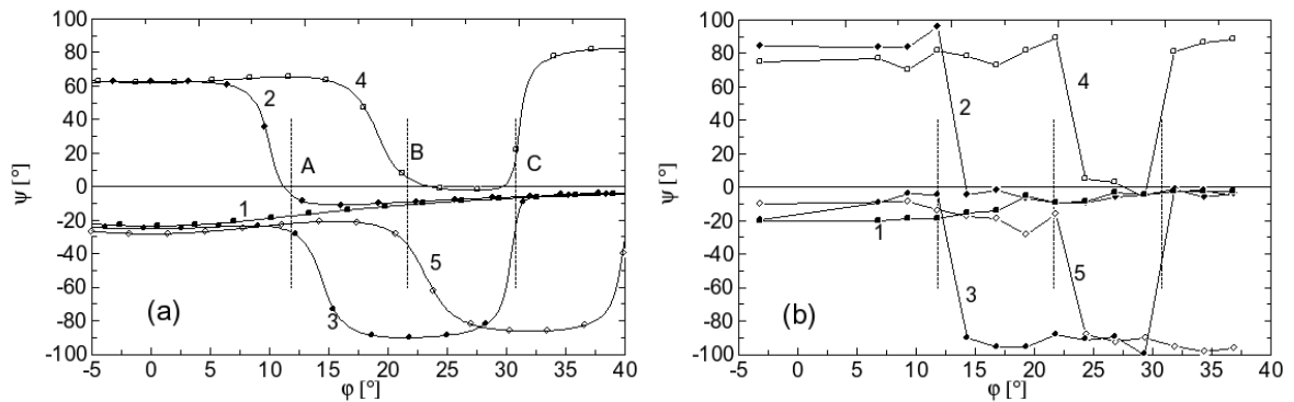
Fig. 4 : Variation de l'angle de polarisation \psi des modes reportés sur la figure 3 en fonction de l'angle de propagation \phi : (a) courbes théoriques, (b) résultats expérimentaux.
