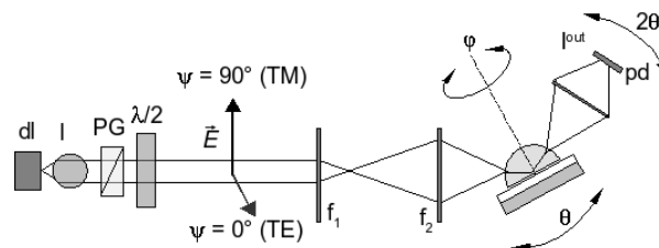
Fig. 2 : Schéma du banc de m -lines hémisphériques (dl: diode laser, l: lentille, PG: prisme de Glan, pd: photo-diode)
