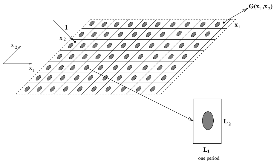
Fig. 2. Periodic medium.
