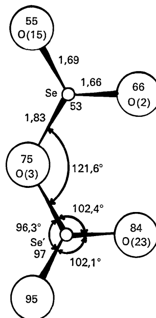
Fig. 2. Groupement (Se_2O_5)^{2-} .
