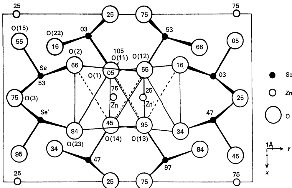
Fig. 1. Projection de la structure de \text{ZnSe}_2\text{O}_5 sur le plan (001).
