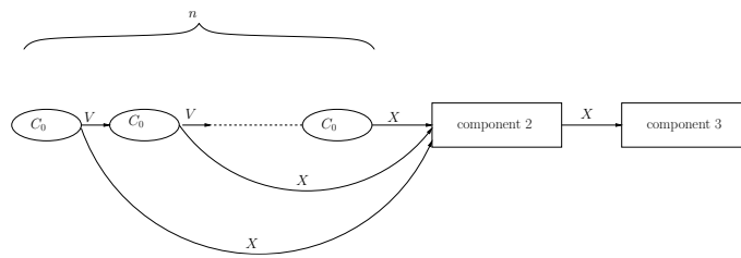
Fig. 7. the automaton T
