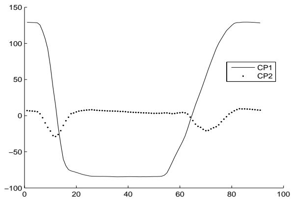
FIG. 4 – Graphe des deux premières CP d’une ACPR ( \theta = 5 ) sur des variables obtenues en enregistrant les coordonnées des membres d’un danseur (mouvement Chute Pliée)
