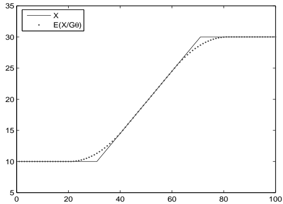
FIG. 3 – Graphe d’une série temporelle X avec son espérance relationnelle E(X|G_\theta) ( \theta = 10 )
