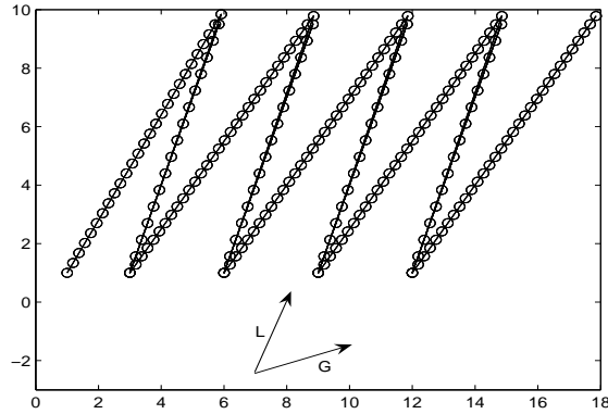
FIG. 2 – Disposition des individus (petits cercles) avec deux vecteurs propres : l’un issu d’une ACP standard (G) et l’autre d’une ACPR (L) avec \theta = 5
