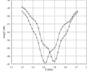
FIG. 2 – Amplitude de \Gamma ( \text{Amp}(\Gamma) , unité : dB) en fonction de la fréquence ( F , unité : GHz), o : circuit "type 0°", + : circuit "type 90°".
