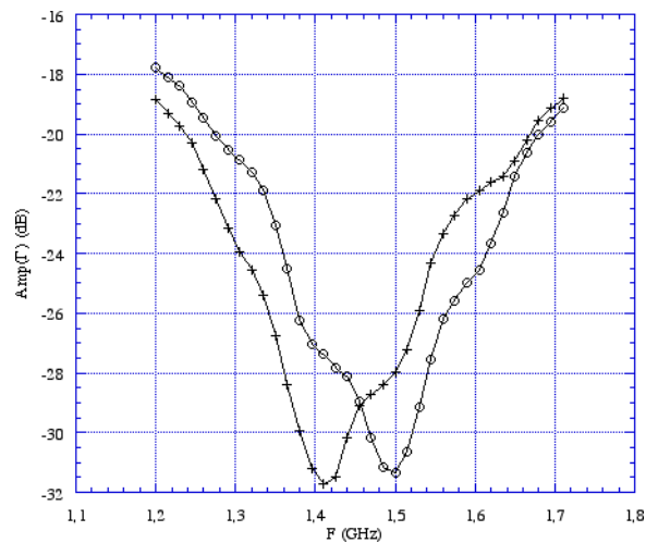
Figure 2. Amplitude de \Gamma ( Amp(\Gamma) , unité : dB) en fonction de la fréquence ( F , unité : GHz), o : circuit "type 0°", + : circuit "type 90°"
