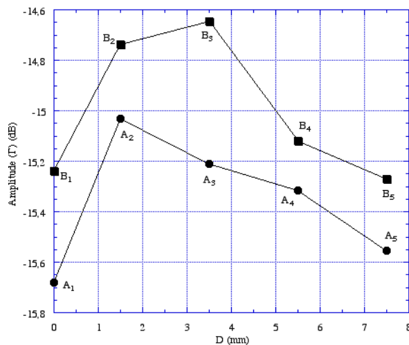
Figure 7. Amplitude du coefficient de réflexion (Amplitude \Gamma ), unité : dB en fonction du déplacement maximum atteint ( D , unité : mm) aux points ( A_{i=1,\dots,5} ) sans charge et ( B_{i=1,\dots,5} ) sous charge (figure 5) (Mesures à 2 GHz).
