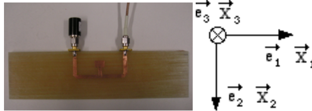
Figure 4. Instrumentation de l'éprouvette (vue de la peau inférieure)
