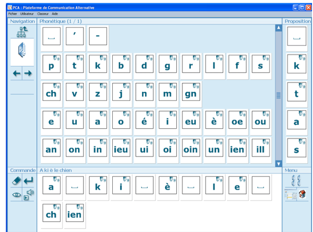
Figure 7. Clavier phonétique
