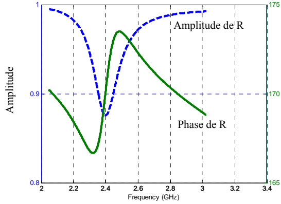
Fig. 5: Exemple d'une SSR combinée donnant une augmentation de phase du coefficient de réflexion
