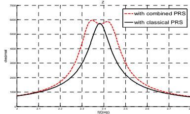
Fig. 7: Comparaison des modules d'impédance
