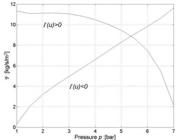
Fig. 7 Function \Psi .
