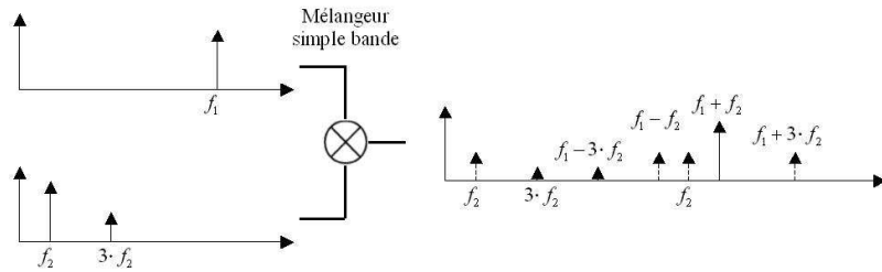
Figure 4 : Spectre à la sortie du mélangeur simple bande.
