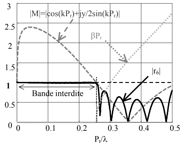
Figure 10 : Structure périodique à six couches, coefficient de réflexion et module de M (6). ( a=1\text{mm} , P_r=C_1=40\text{mm} , P_\alpha=60^\circ/i ( i=1,2,\dots ), P_t constant)
