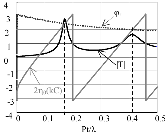
Figure 6 : Confirmation que les points d'intersections de \phi_r et 2\eta_0(kC) correspondent aux pics de |T| ( a=2mm , P_\theta=30^\circ , P_t=200mm \cdot \pi/6 \approx 105mm )
