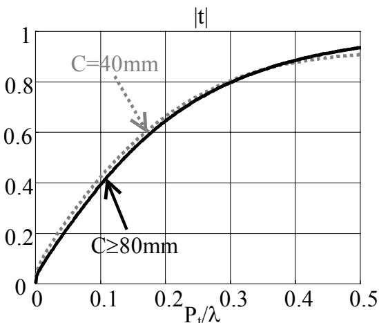
Figure 7 : Module de t pour une structure périodique de tiges métalliques pour différentes valeurs de C , ( a=1mm , P_t=\pi/6 \cdot 40mm constant).
