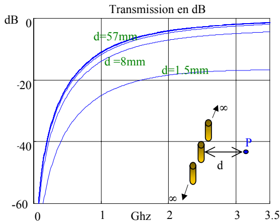
Fig. 2a : courbe de transmission d'une couche infini pour différentes positions du point d'observation. Point d'observation en face d'une tige
