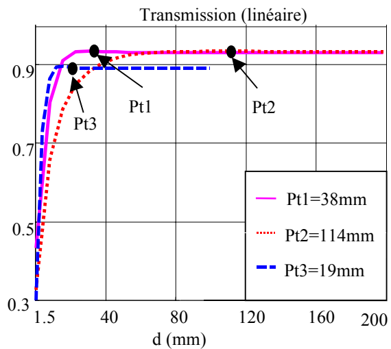
Fig. 4b : transmission en fonction de la distance d pour différentes périodes Pt. (a=1mm)
