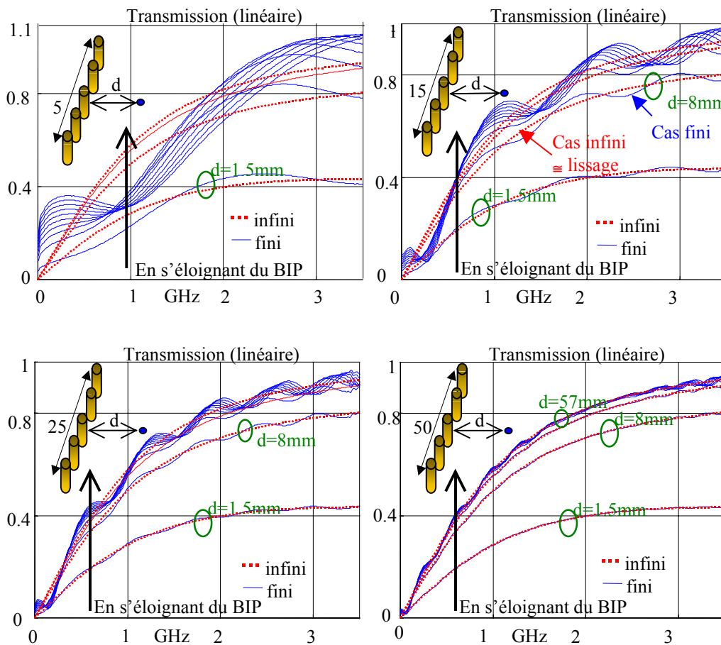
Fig. 5 : coefficient de transmission d'une couche fini pour différents nombres de tiges. Lorsqu'on augmente le nombre de tiges, les courbes tendent vers le résultat du cas infini représenté en pointillé pour 4 points d'observation (le premier point d'observation étant à 0.5mm d'une tige et le dernier à une période et demi)
