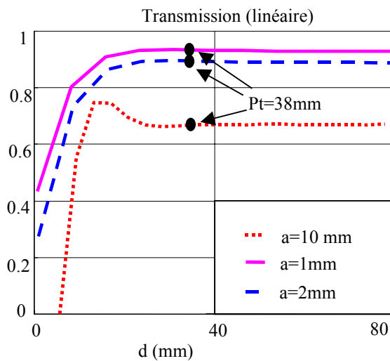
Fig. 4a: transmission en fonction de la distance d pour différents diamètres des tiges a. (Pt=38mm)
