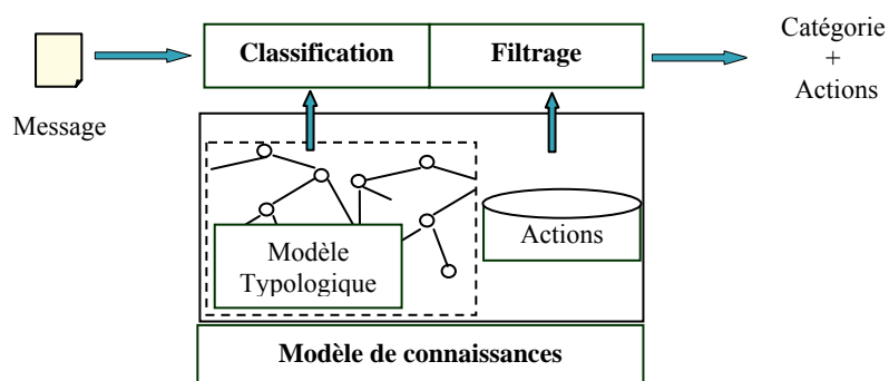
Figure 3. Processus de classification et de filtrage
