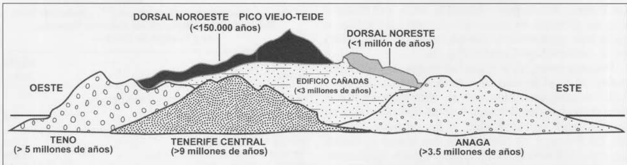
Fig. 2.—La isla de Tenerife emergió hace unos 12 millones de años y se construyó por el apilamiento de tres grandes volcanes en escudo —Tenerife central, Teno y Anaga (Carracedo, 1979; Guillou et al. , 2004a). A este período de intenso volcanismo le sucedió un largo período de reposo (similar al que ahora experimenta La Gomera), tras el cual se levantó en su centro el edificio volcánico Cañadas, que colapsó hace cientos de miles de años para formar la caldera de su nombre. La última etapa eruptiva, y la única que interesa a efectos de definir el riesgo volcánico de Tenerife son las dorsales y su consecuencia, el edificio central Teide.
