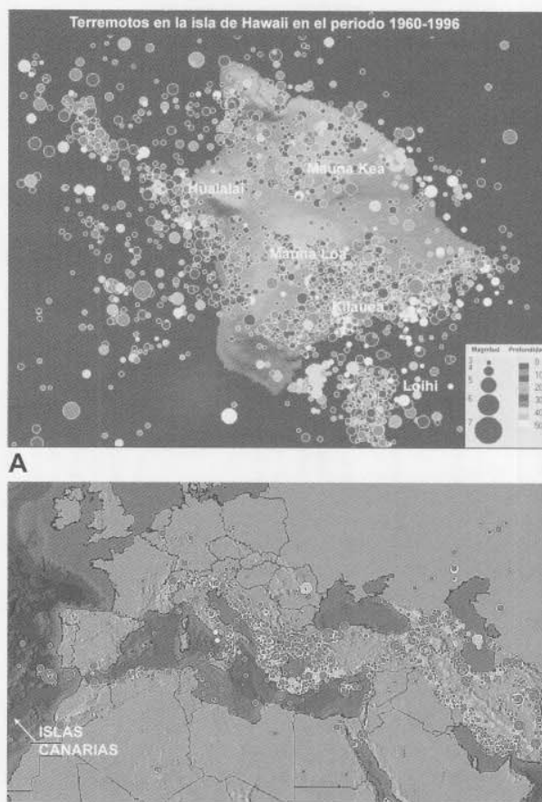
Fig. 7.—A) Terremotos de magnitud >3 registrados en la isla de Hawaii en el período 1960-1996. La mayoría son de 5-6 grados de magnitud, pero se han superado los 7. Como puede observarse son todos volcánicos, relacionados con los volcanes activos, incluyendo los de los flancos submarinos, como el volcán submarino Loihi, la próxima isla que emergerá. B) Sismicidad ( M > 5 ) registrada en el Atlántico Norte, Europa y el norte de África en el período 1960-2003. Obsérvese la escasa incidencia en las Islas Canarias, archipiélago volcánico oceánico situado en el interior de la Placa Africana, en comparación con las zonas circundantes de borde de placa (Imágenes tomadas de Earthquakes and Eruptions, de la Smithsonian Institution Global Volcanism Program, www.volcano.si.edu/gvp/ ).
