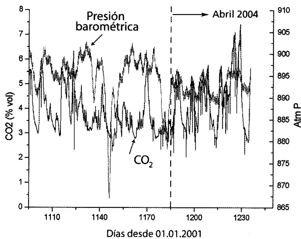
Fig. 9.—Modulación de la tasa de emisión de CO 2 por los cambios de corto período y estacionales de la presión barométrica. Puede observarse la falta de cambios significativos asociados a la sismicidad de abril-mayo de 2004 (com. pers. C. Martín).
