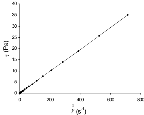
Figure 1 : Comportement rhéologique de l'additif
