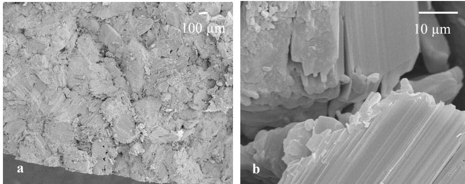
Photo 3. Faciès de rupture de comprimés réalisés à 60 °C.
