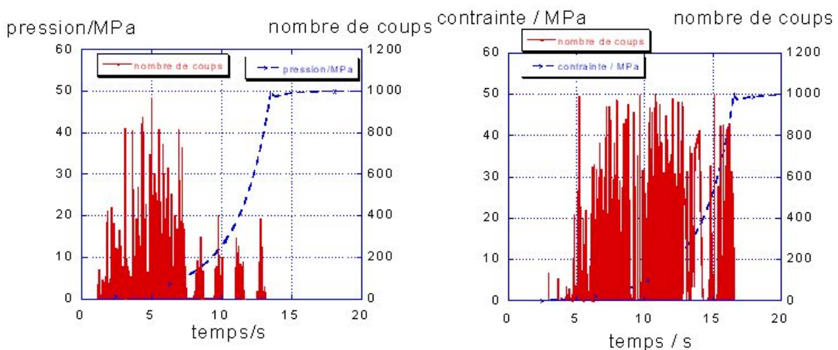
Figure 5. Courbes de pression et d'EA en fonction du temps pour le produit A à 25°C (gauche) et à 40°C (droite).
