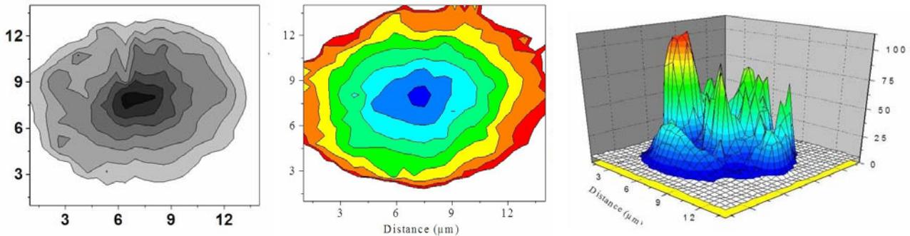
Figure 10: Images Raman montrant (a) l'hétérogénéité de concentration en seconde phase de carbone (concentration maximale au cœur) et (b) la différence d'aromaticité du carbone ( faible aromaticité au cœur) au travers d'une section d'une fibre SiC SA3 (Ube Industry, Japon); L'image Rayleigh en c) montre l'implication des ces hétérogénéités sur la corrosivité par des sels alcalins. Reproduit avec l'autorisation de Wiley (C) 2003, Spectroscopy Europe 15, 8.
