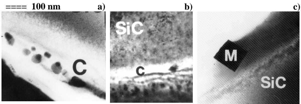
Figure 3 : Microphotographies des interfaces SiC Nicalon NLM202 (Nippon Carbon, Japon) avec des matrices de type a) LAS, b) CAS et c) mullite "vitreuse" ( le carré noir est un cristal de mullite). Noter dans les cas a) et b) la présence d'une interphase de carbone, apparaissant en blanc et son absence en c); la fibre SiC est au-dessus, les matrices, en bas. Reproduit avec l'autorisation des Editions de Physique, © 1993, J. Physique C-7 , 1937, ibidem 1941.
