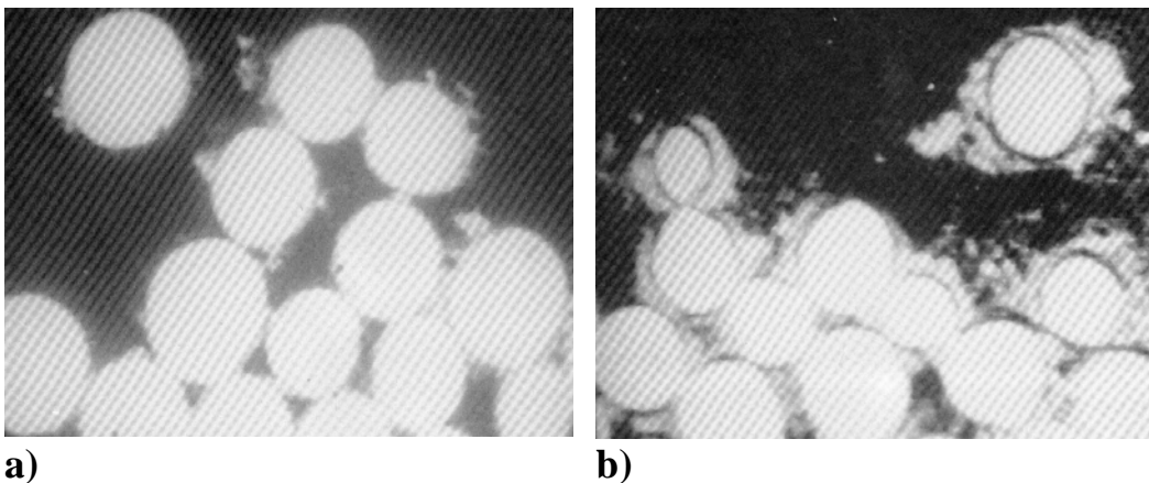
Figure 4 : Images EDX de la concentration en élément Si pour des sections de composites fibres SiC Nicalon NLM202-matrice \text{Al}_2\text{TiO}_5 préparés par pressage à chaud à 1270°C (a) et 1350°C (b). Noter la diffusion importante des atomes de silicium en b). Diamètre des fibres \sim 12 \mu\text{m} . Reproduit avec l'autorisation de l'AMAC, Proc. 8 ème Journées Nationales sur les Composites, JNC'8, 16-18 novembre 1992, Palaiseau, O. Allix, J.P. Favre et P. Ladevèze eds., AMAC, Paris (1992) p. 253-264.
