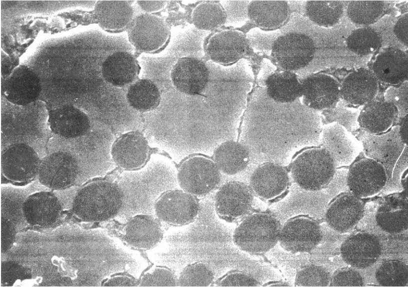
Figure 2 : Exemple de fissuration matricielle provoquée par la densification de la matrice à l'intérieur d'une structure fibreuse restant invariante géométriquement.
