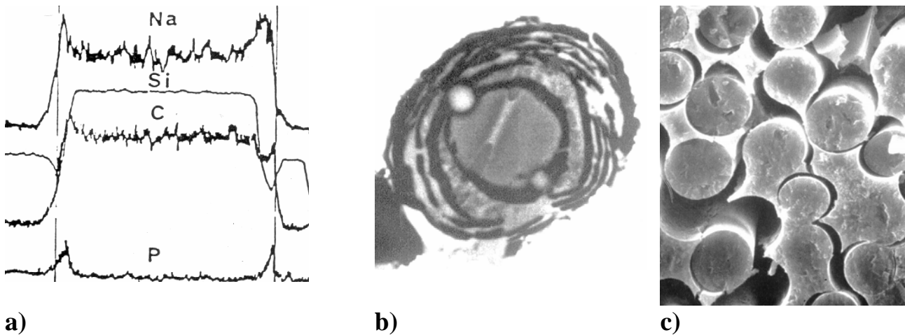
Figure 5 : Profils EDX de concentration des éléments Na, Si, C et P au travers d'une fibre Nicalon NLM 202 dans une matrice riche en sodium (a); noter l'interface de carbone enrichie en sodium et phosphore se formant à l'interface fibre-matrice. Dans certains cas la réaction permet de visualiser l'hétérogénéité de réactivité (c.a.d. de composition) des fibres. La bonne dé-cohésion fibre-matrice de ce type d'interface est montrée sur une section polie d'un composite fibre SiC-matrice NASICON après rupture en flexion (d'après ref [28]).
