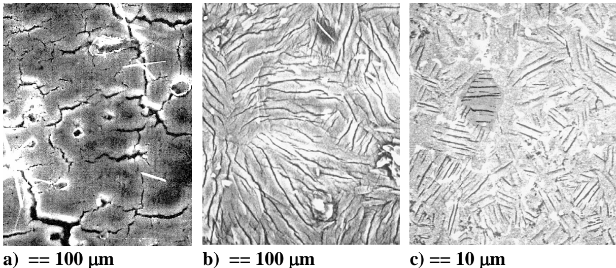
Figure 6 : Micrographies visualisant les fissures se produisant pour des sections polies de LAS ( a) amorphe, c) cristallisé en \beta spodumène et b) état intermédiaire) après attaque pendant 0.5 h par H_2SO_4 concentré à ébullition, traitement simulant bien l'attaque par les protons pendant un cycle de combustion d'une turbine.
