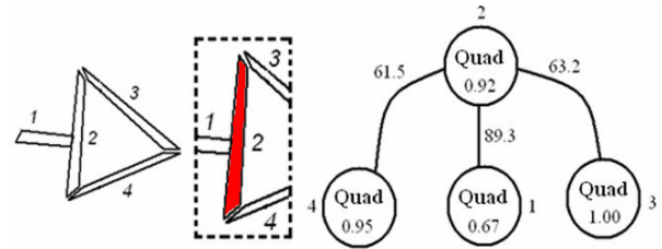
FIG. 4 - Partie du graphe associé au quadrilatère 2
