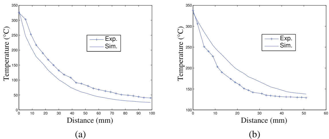
Figure 3. Comparaison essais-simulation : (a) comparaison sur la ligne située en amont de l'outil (b) comparaison sur la ligne perpendiculaire au trajet de l'outil
