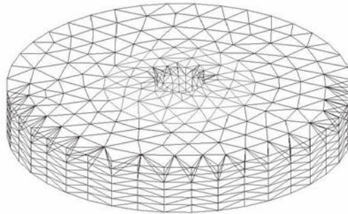
Figure 5. Domaine cylindrique réduit utilisé pour le calcul de l'écoulement autour de l'outil
