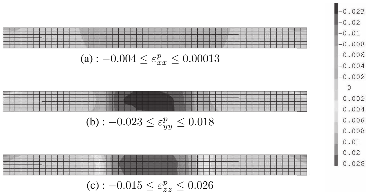
Figure 6. Écoulement de la matière autour de l'outil pour différentes hauteurs (seul le pion est représenté) : (a) un quart de l'épaisseur des plaques (b) la moitié de l'épaisseur des plaques (c) trois quarts de l'épaisseur des plaques
