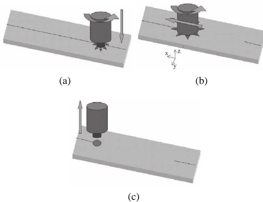
Figure 1. Description du Friction Stir Welding : (a) plongée de l'outil dans les plaques (b) avancement de l'outil en rotation (c) retrait de l'outil
