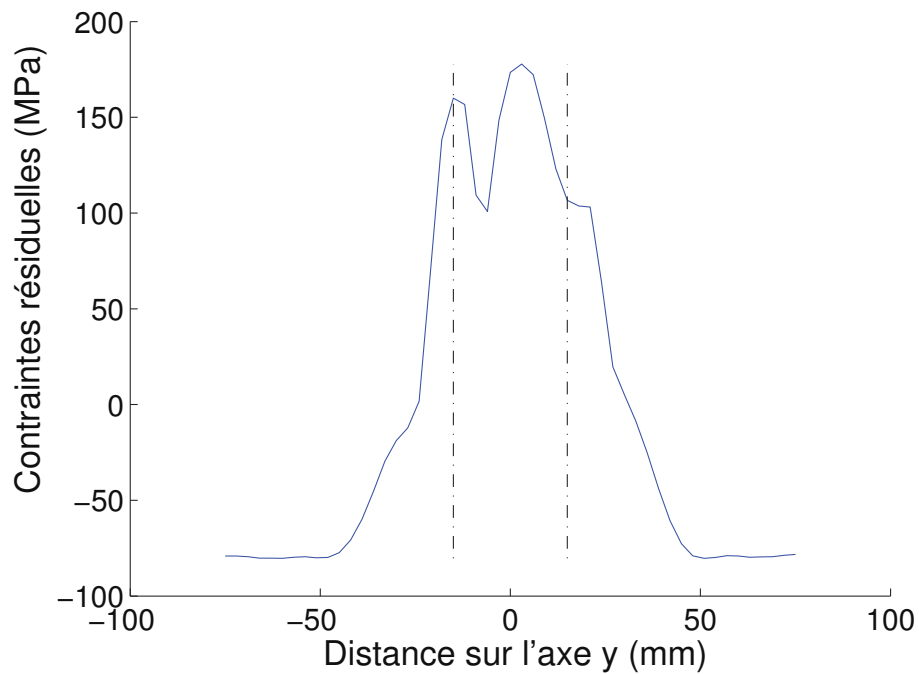
Figure 9. Profil de la composante \sigma_{xx}^{res} le long d'une ligne transversale située à mi-hauteur des plaques. Les lignes pointillées correspondent au rayon de l'épaulement et le point x = 0 correspond à la ligne centrale.
