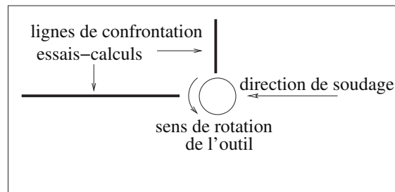
Figure 2. Représentation schématique des deux lignes permettant de confronter calculs numériques et essais expérimentaux
