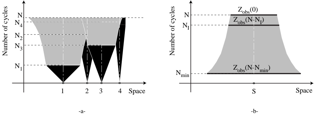
Figure 1. -a-Depiction of two mesocrack propagations (1 and 3) and obscuration for two microcracks (2 and 4). -b-Horizon for a given location S. -a-Schématisation de la propagation de deux mésocraques (1 et 3) et de l'écrantage de deux microfissures (2 et 4). -b-Horizon en un lieu donné S.
