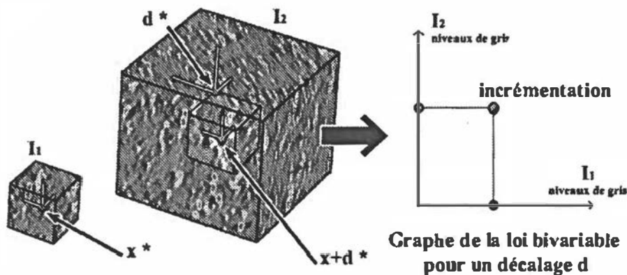
Figure 20. Création du graphe de la loi bivariable pour un décalage d et un voxel x
