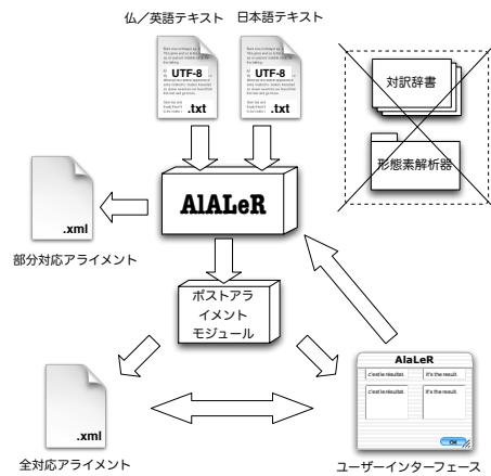
図 1 システム『あられ』
