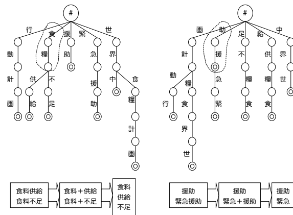
図3 前接(図左)・後接(図右)部分文字列検出用トライ
