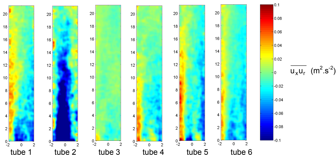
Fig. 14 Covariance des fluctuations de vitesse axiale et radiale pour le débit d'entrée de 12 l.min -1
