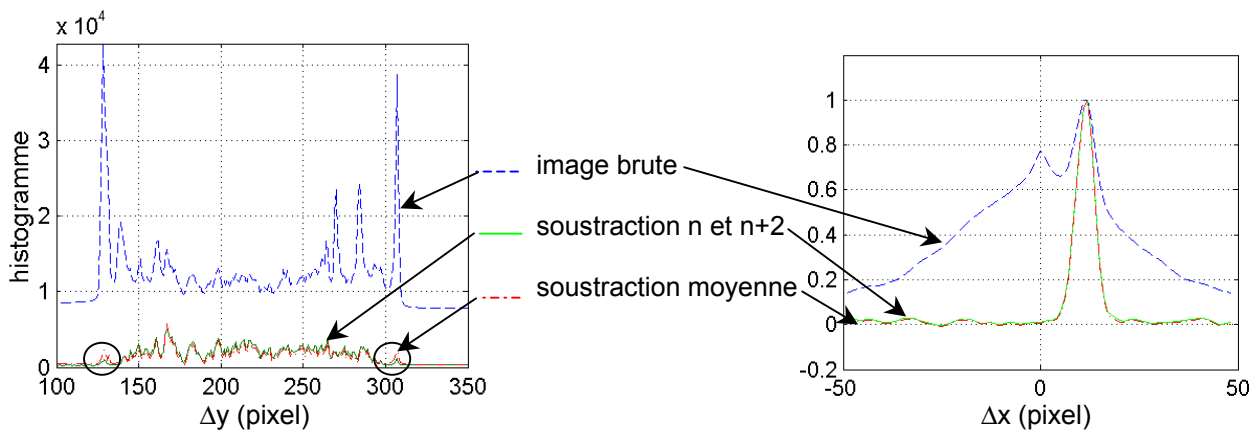
Fig. 6 Histogramme de l'image brute, avec soustraction du bruit de fond moyen et avec soustraction des images n et n+2 (à gauche) et intercorrélation en \Delta y = 0 pour une paire de ces mêmes images (à droite)
