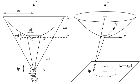
FIG. 4 – À gauche : notation utile (et abrégées) pour l'estimation de z^p et f^p . À droite : t^p est située sur un cercle dans le plan z = -z^p étant donné \frac{z}{z^p} et l'angle entre la direction de t^p vers les centres des grands et petit cercles.
