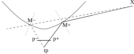
FIG. 3 – Le rayon qui passe par un point X et le centre de la caméra perspective t^p est réfléchi par le miroir en un point M^+(t^p, X) et est projeté par la caméra perspective en p^+(X) . On définit aussi le point M^-(t^p, X) sur le miroir, projeté en p^-(X) . M^-(t^p, X) est comme M^+(t^p, X) , à ceci près que le rayon réfléchi de M^-(t^p, X) vers X pointe vers l'intérieur du miroir, pas l'extérieur. Les points M^+(t^p, X), p^+(X), M^-(t^p, X), p^-(X) sont abrégés M^+, p^+, M^-, p^- dans cette figure. On note que X, M^-, M^+ ne sont pas nécessairement alignés.
