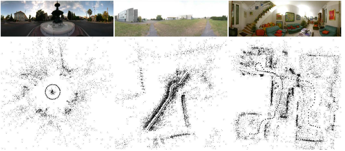
FIG. 6 – En haut : panoramiques obtenus à partir d’une image de chaque séquence. En bas : vues de dessus des reconstructions 3D avec la position des caméras (petits carrés) et des points 3D (points noirs). À gauche : Fontaine (38 vues, 5857 points). Au milieu : Chemin (54 vues, 10178 points). À droite : Maison (112 vues, 15504 points). Certains de ces points sont difficiles à reconstruire lorsqu’ils sont alignés (ou presque) avec les caméras à partir desquelles ils sont reconstruits. Ces résultats sont similaires pour les caméras à centre unique (avec une fonction r(\alpha) affine ou cubique) ou à centre non-unique.
