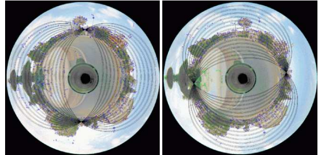
FIG. 7 – Courbes epipolaires pour la géométrie de deux paires d’images différentes de la séquence Fontaine. Les deux epipoles à gauche sont cohérents avec le véritable mouvement de la caméra autour de la fontaine car ils indiquent la direction du mouvement de la caméra. Ce n’est pas le cas pour ceux de droite, et de telles erreurs sont corrigées par les ajustements de faisceaux.
