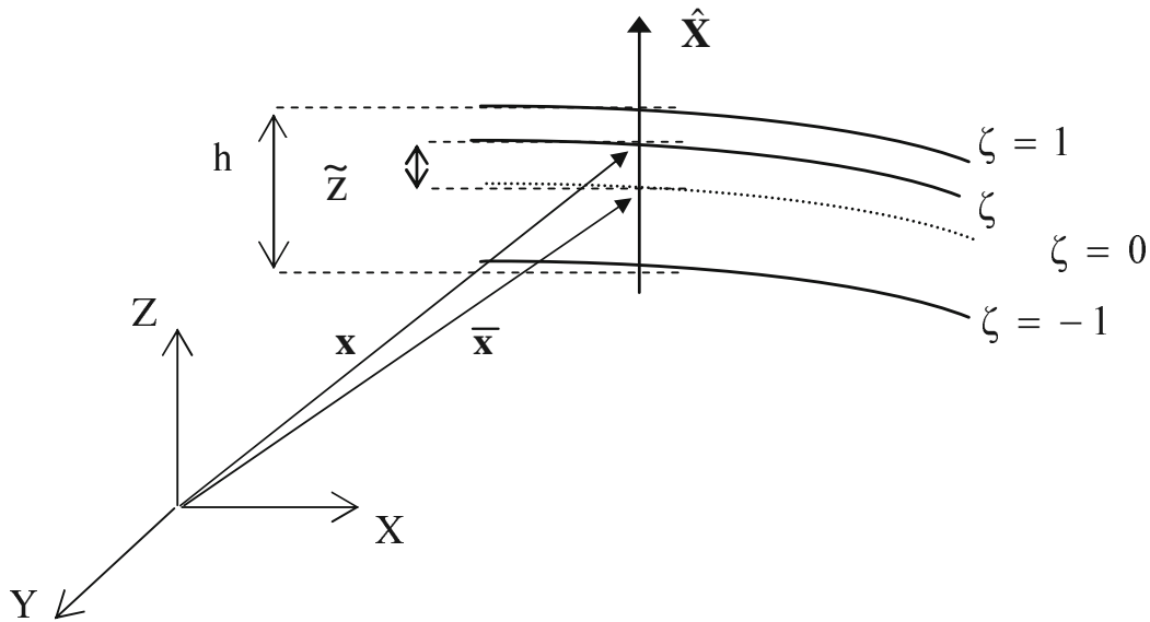
Figure 5. Géométrie de la coque
