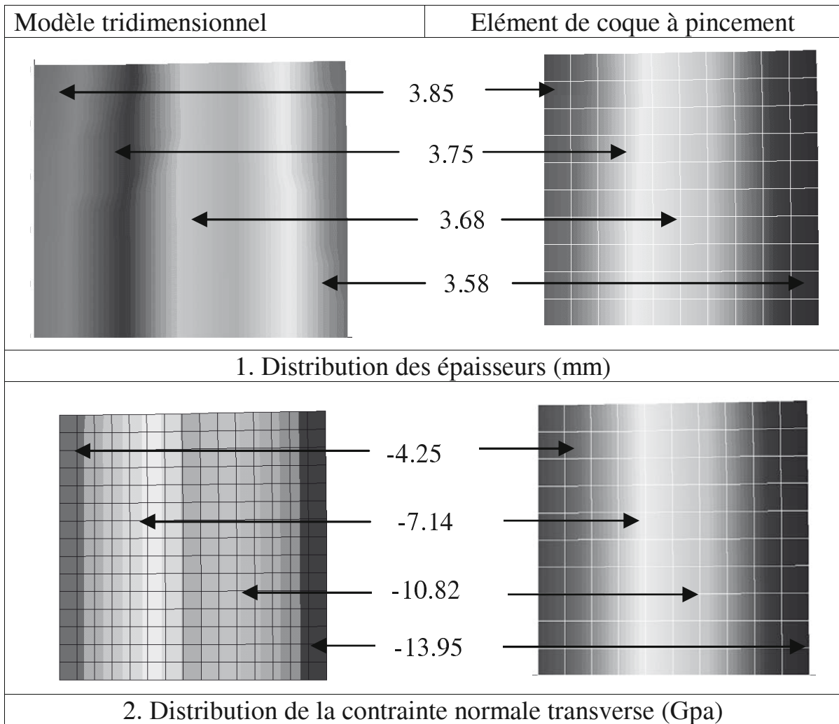
Figure 14. Comparaison coque à pincement – tridimensionnel
