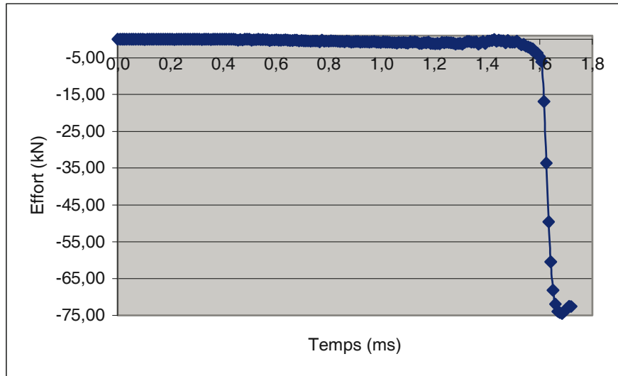
Figure 23. Effort de contact lors du processus
