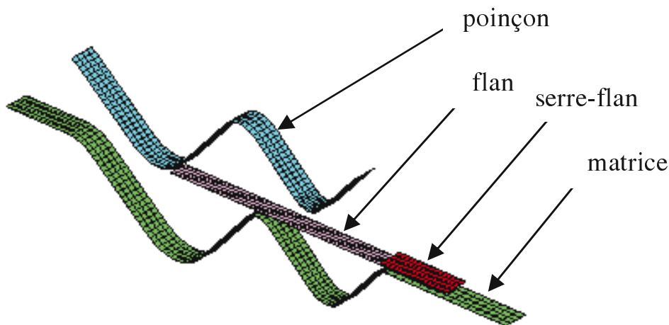
Figure 20. Maillage à l'état initial
