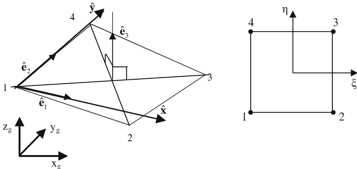
Figure 7. Définition des repères et élément de référence à quatre nœuds associé
