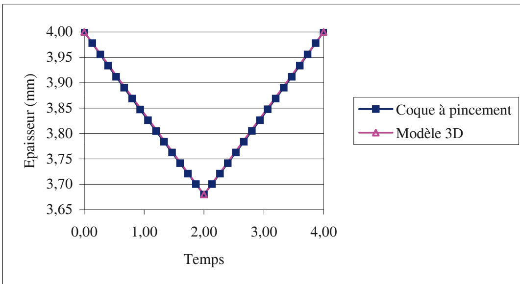
Figure 12. Evolution de l'épaisseur
