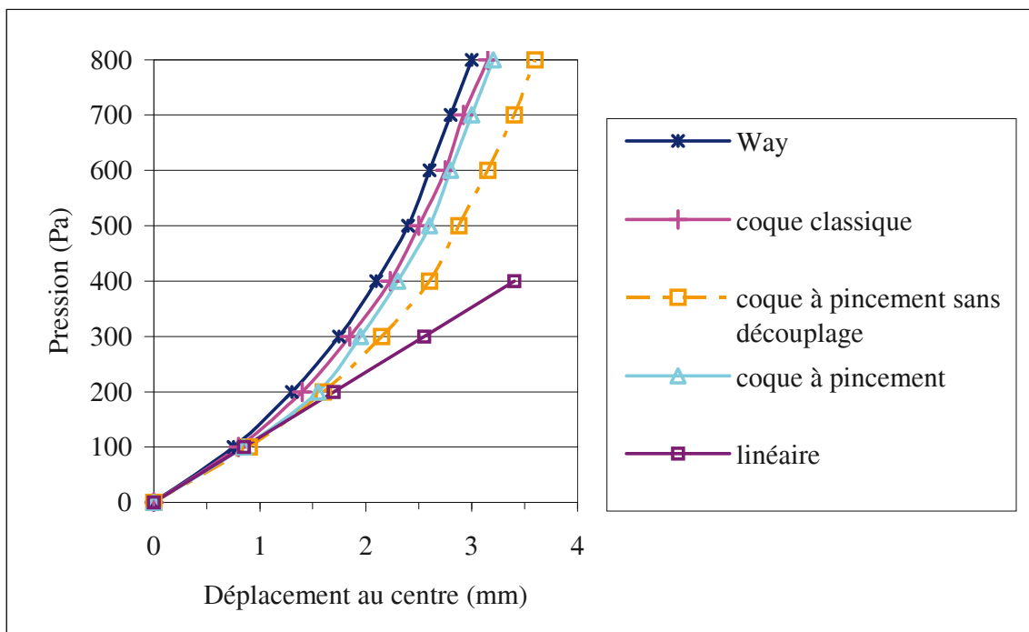
Figure 17. Déplacement au centre de la plaque
