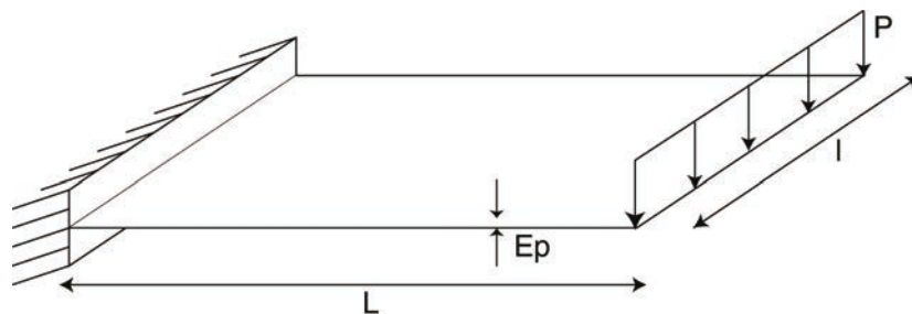
Figure 9. Poutre console en flexion
