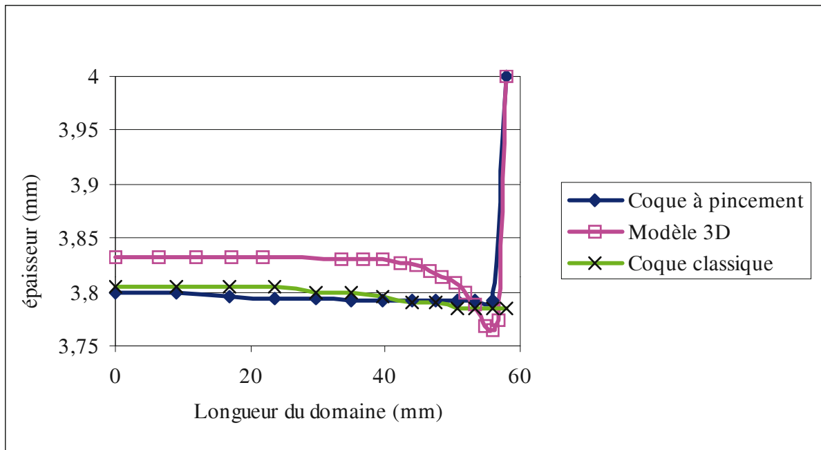
Figure 15. Variation d'épaisseur pour les 3 modèles
