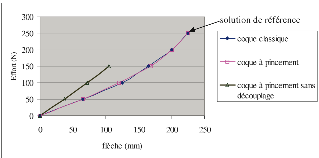
Figure 18. Comparaison des différents modèles. Poutre console
