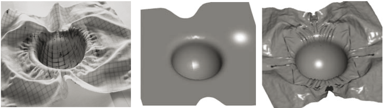
Figure 4. Emboutissage hémisphérique d'un tissu très déséquilibré
