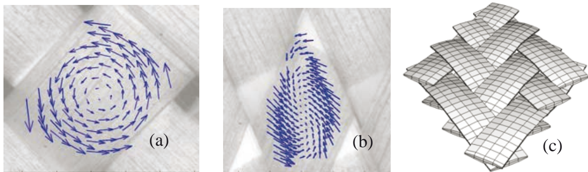
Figure 2. Champ de déplacement dans la mèche avant (a) et après (b) le blocage. (c) Analyse par éléments finis 3D
