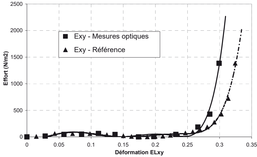
Figure 3. Courbe d'effort dû au cisaillement plan
