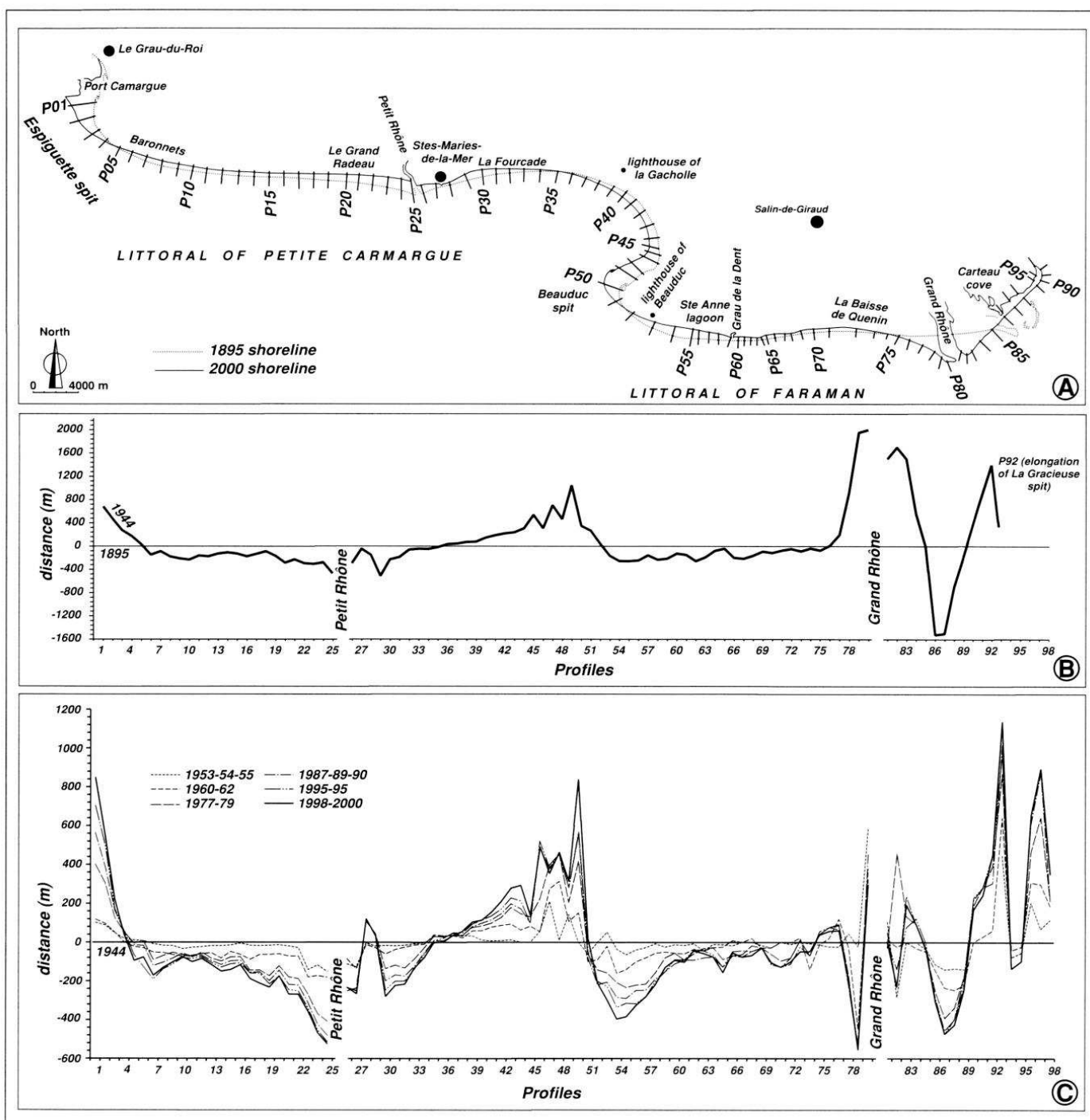
Fig. 5 – Variations du trait de côte entre 1895 et 2000. A : position des profils ; B : variations du trait de côte entre 1895 et 1944 ; C : variations du trait de côte entre 1944 et 2000.
