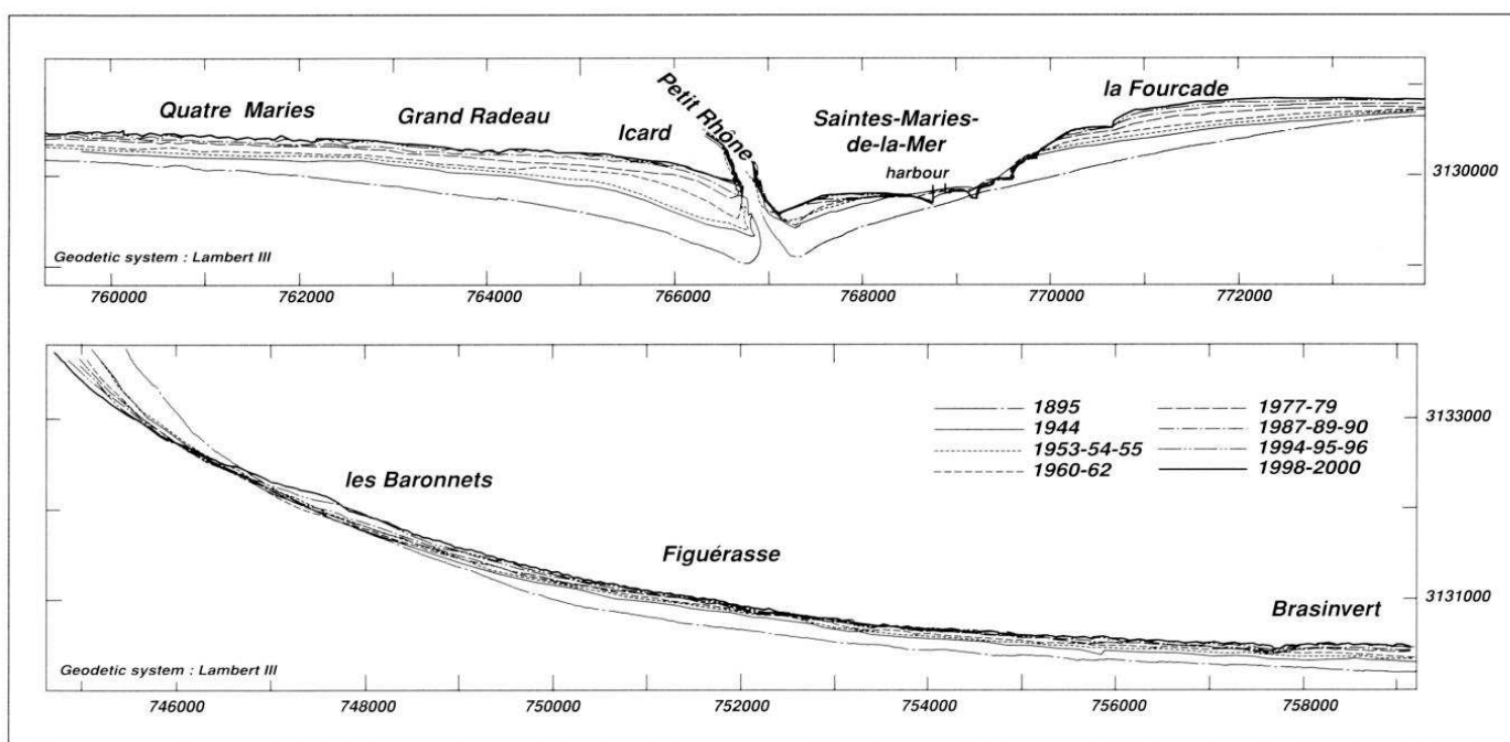
Fig. 9 – Variations du trait de côte du littoral des Saintes-Maries-de-la-Mer et de la Petite Camargue entre 1895 et 2000.
