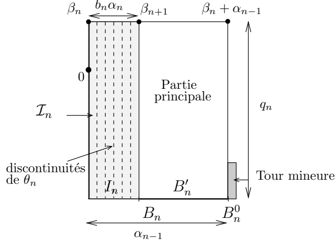
Fig. 5 – Les tours de \mathcal{D}_n(\beta) .
