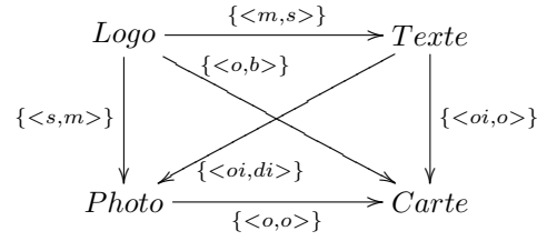
FIG. 6 – Graphe de relations directionnelles de la spécification de la Figure 2.
