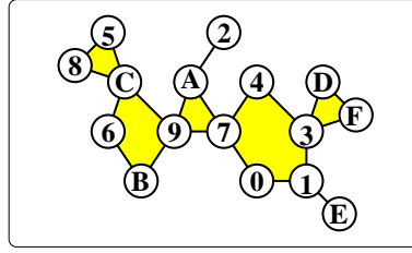
FIG. 1 – Un exemple d’hyperarborescence sur \{0, 1, 2, 3, 4, 5, 6, 7, 8, 9, A, B, C, D, E, F\} .
