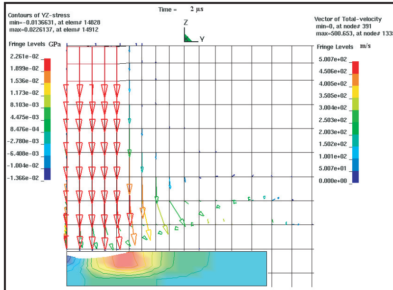
Fig. 11. Distribution des contraintes de von Mises (YZ) et du champ de vitesse fluide visualisé dans la section transversale (A1-A2) (temps = 2 \mu\text{s} ).
