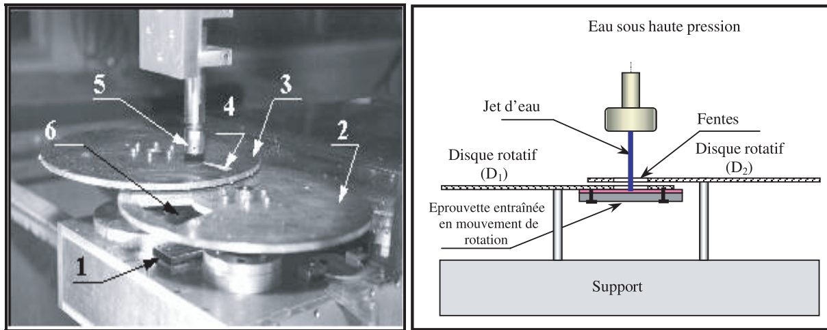
Fig. 20. Montage expérimental de mesure du temps d'exposition d'une cible à un jet d'eau HP (éprouvette (1), disques rotatifs (2, 3), buse (5), fentes (4, 6)).
