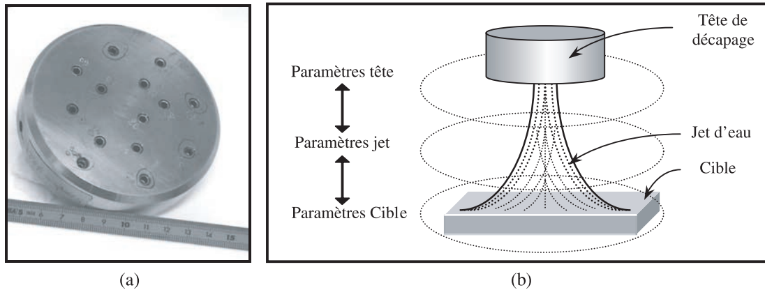
Fig. 1. (a) Tête multi-buses de décapage. (b) Paramètres de décapage.
