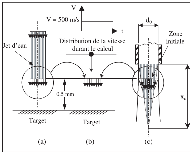
Fig. 3. (a) Jet cylindrique : cas du modèle numérique. (b) Vitesse introduite dans la modélisation. (c) Structure d'un jet accéléré : cas réel.
