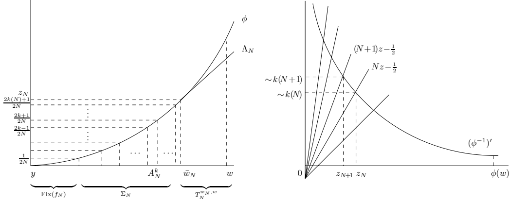
FIG. 1 – Représentation de T_N(f) et construction de la suite k(N) associée.
