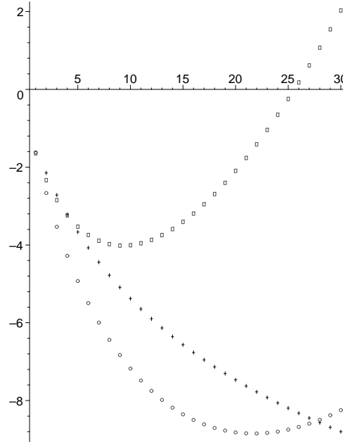
FIGURE 2. Nous avons représenté pour A = B = 1 , z = 10 + 10i et n = 0, \dots, 30 , par \square les points de coordonnées [n, \log |R_{as}(\ln(2), 1, 1, n, z)|] , par \circ les points de coordonnées [n, \log |R_{as}(\frac{\pi}{2}, 1, 1, n, z)|] , par + les points de coordonnées [n, \log |R_{fact}(1, 1, 1, n, z)|] .
