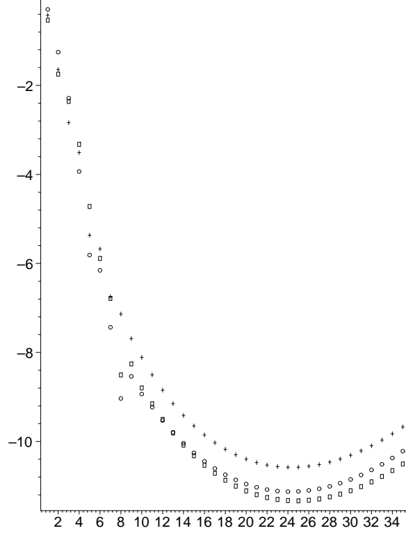
FIGURE 3. Nous avons représenté pour z = 12 et j = 1, \dots, 35 , par \square les points de coordonnées [j, \log |\frac{a_{1,j}}{z^j}|] , par \circ les points de coordonnées [j, \log |\frac{a_{2,j}}{z^j}|] , par + les points de coordonnées [j, \log |\frac{a_{3,j}}{z^j}|] .
