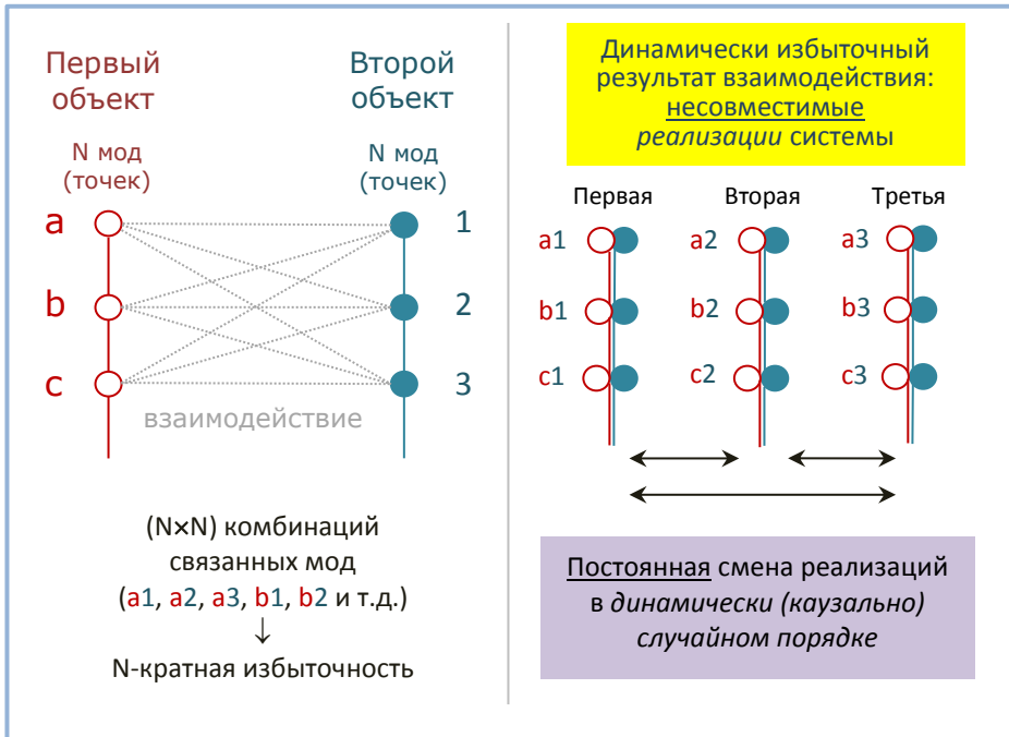
Рис. 2. Возникновение динамической многозначности в любом реальном процессе взаимодействия. Передурцированное взаимодействие между двумя объектами (например протополями) с N взаимодействующими точками или модами каждый (слева) даёт N^2 комбинаций мод, что ведёт к N -кратной избыточности образовавшихся таким образом несовместимых реализаций системы (в соответствии с уравнениями (6), (11)). Она связана с симметрией сложности, ибо “число мест” для компонент и продуктов взаимодействия, определяемое полной сложностью системы, не может измениться в процессе взаимодействия. Поэтому все N_{\text{эР}} = N одинаково реальных реализаций системы вынуждены, под действием того же движущего взаимодействия, постоянно замещать друг друга в определённом таким образом динамически случайном порядке (справа).
