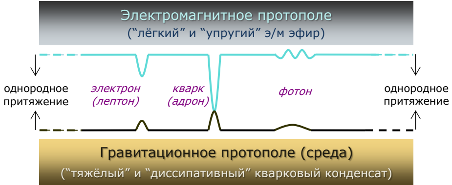
Рис. 1. Схема конфигурации и развития нередуцированного взаимодействия протополей, приводящего к динамическому возникновению (последовательно выводимых) элементарных частиц, полей, их свойств и взаимодействий.
