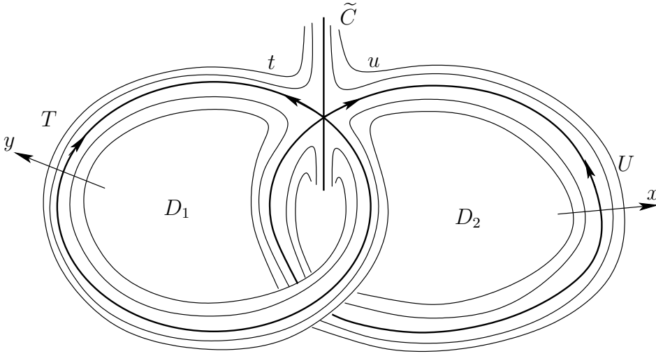
FIGURE 4. Deuxième éclatement du cusp
