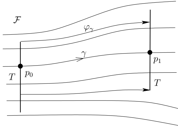
FIGURE 2. Holonomie d'un chemin entre deux transversales
