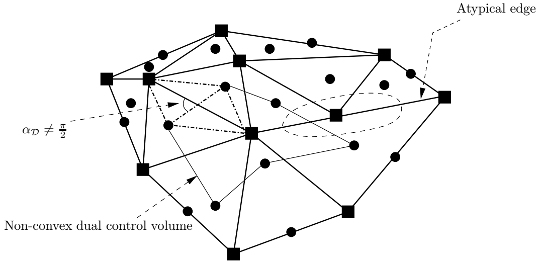
FIG. 2.3. Non conformal meshes
