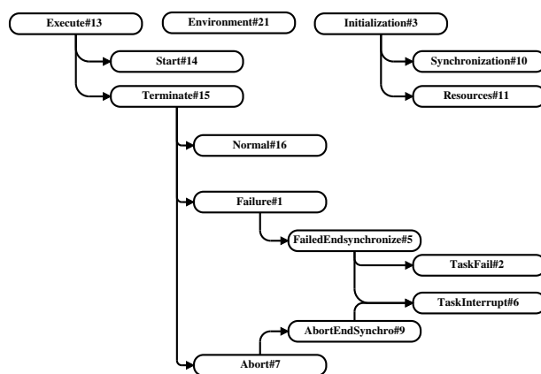
FIG. 7 – La hiérarchie initiale du modèle
