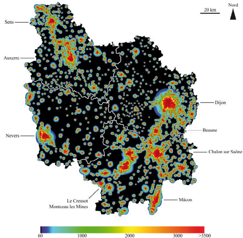
Figure 1 : modélisation cartographique de la luminance du ciel au zénith (en nanoLamberts, nL , 60 nL correspondant à la luminosité naturelle du ciel nocturne) en Bourgogne, à partir des données de population INSEE (RGP 1999) et des données d'occupation du sol Corine Land Cover (2000). Modèle : Albers et Duriscoe (2001). Cartographie : Samuel Challéat, Théma Université de Bourgogne.
