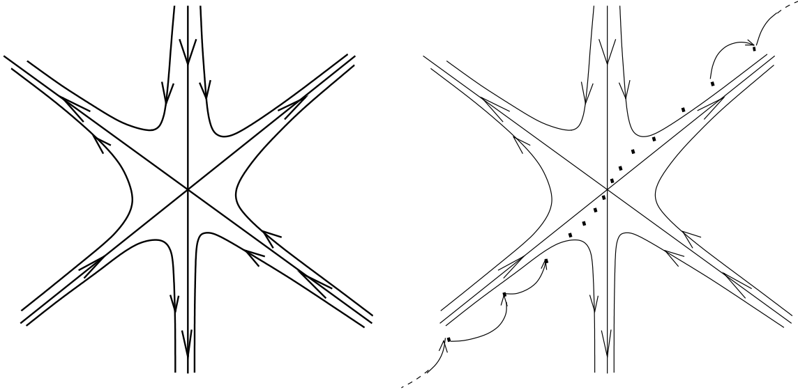
FIGURE 1 – Exemple de point fixe non contournable. La pseudo-orbite de la figure de droite ne peut pas être remplacée par une orbite ayant les mêmes entrée et sortie dans le voisinage du point fixe.
