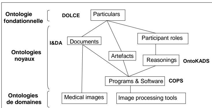
Fig. 1 – Structure de l'ontologie d'application du projet NeuroLOG
