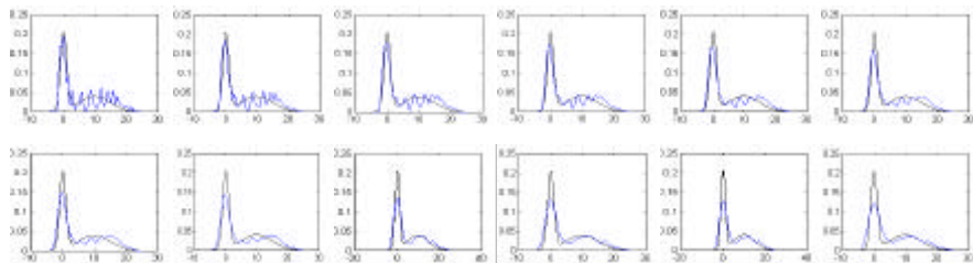
Figure 2: Densité multi-modale avec hétérogénéité de dispersion et taille de fenêtre unique on n'estime jamais les deux composantes à la fois
