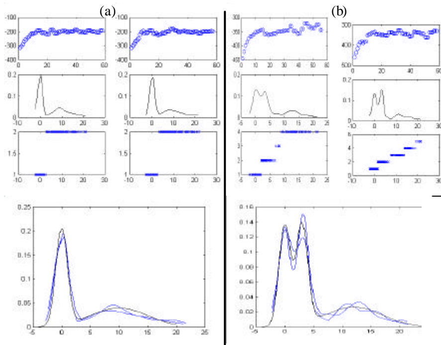
Figure 4 : Quelques résultats (a) : 200 points tirés pour moitié sur \mathcal{N}(0,1) et pour moitié sur \mathcal{N}(10,5) 2 exemples (pseudo-vraisemblance, estimation de densité et segmentation) et comparaison de la densité estimée à la vraie densité. (b) 300 points tirés pour tiers sur \mathcal{N}(0,1) , pour tiers sur \mathcal{N}(3,1) et pour tiers sur \mathcal{N}(12,5)
