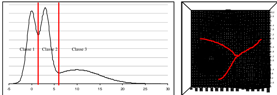
Figure 1 : classification sous hypothèse de densité connue
