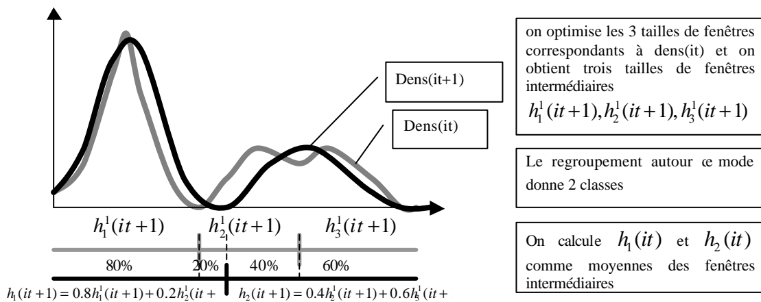
Figure 3 : Etapes de l'algorithme
