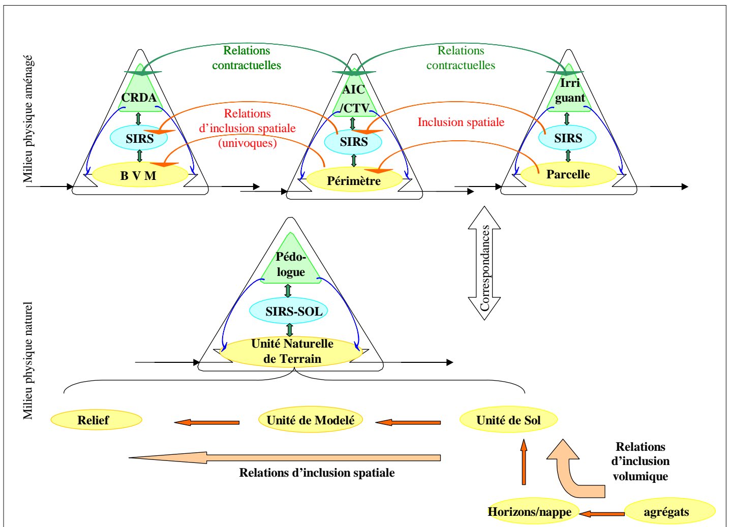
Figure 4. Les deux types de modèles du milieu hydro-agricole isomorphes du système général : les systèmes de gestion ou d'exploitation d'unités spatialisées et les systèmes géomorpho-pédologiques.
