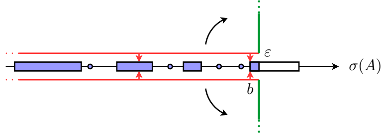
FIGURE 4.4 – Les formules de Stone (4.49) et (4.50) permettent d'exprimer un projecteur spectral sous la forme \mathbb{1}_{]a, b[}(A) comme l'intégrale de la résolvante (A - z)^{-1} sur les droites représentées.
