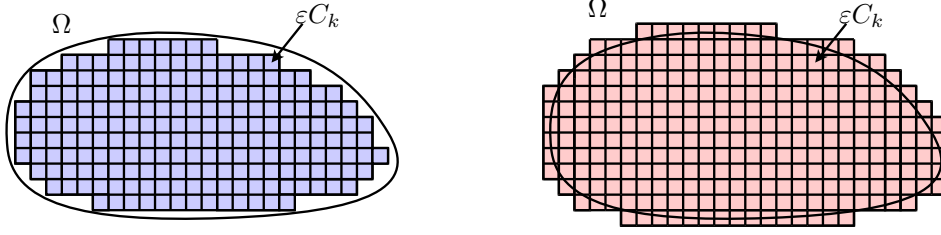
FIGURE 5.5 – Preuve du théorème 5.50 : on utilise les fonctions propres de tous les petits cubes \varepsilon C_k inclus dans l'ouvert \Omega comme fonctions tests pour le Laplacien de Dirichlet sur \Omega , ce qui fournit une borne supérieure sur ses valeurs propres (donc une borne inférieure sur N_{\text{Dir}}(E, \Omega) ). Puis on utilise toutes les fonctions propres des cubes qui intersectent \Omega avec la condition de Neumann, ce qui fournit une borne inférieure sur les valeurs propres dans le domaine \Omega (donc une borne supérieure sur N_{\text{Dir}}(E, \Omega) ).
