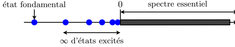
FIGURE 5.2 – Forme du spectre de la réalisation de Friedrichs de l'opérateur de Schrödinger -\Delta + V lorsque V satisfait les hypothèses du théorème 5.47.
