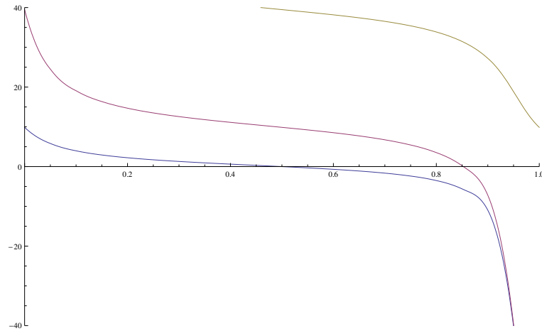
FIGURE 5.6 – Tracé des trois premières valeurs propres \lambda_1(\theta) \leq \lambda_2(\theta) \leq \lambda_3(\theta) du Laplacien de Robin sur l'intervalle ]0, 1[ , en fonction de \theta \in [0, 1[ .
