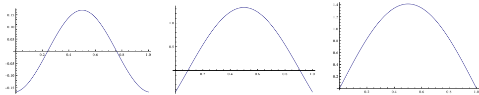
FIGURE 5.7 – Tracé de la troisième fonction propre du Laplacien de Robin sur l'intervalle ]0, 1[ pour \theta = 0.7 , pour \theta = 0.97 et à la limite \theta \rightarrow 1^- .
