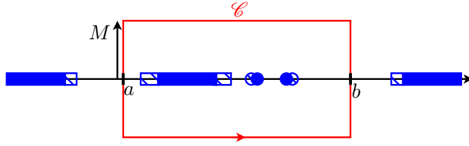
FIGURE 5.1 – Rectangle \mathcal{C} utilisé dans la preuve du théorème 5.2 pour étudier le projecteur spectral P(\varepsilon) = \mathbb{1}_{[a,b]}(A + \varepsilon B) à l'aide de la formule de Cauchy. On prend |\varepsilon| < \varepsilon_0 pour assurer que le spectre de A + \varepsilon B (hachuré sur la figure) reste loin de a et b .
