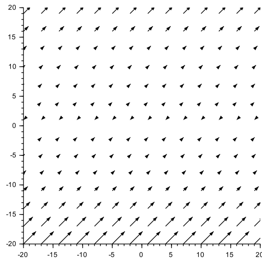
FIGURE 4.1 – La figure montre l'espace de phases de l'équation de Riccati scalaire à coefficients constants suivante \dot{x} = 1 - 4x + 1 .
