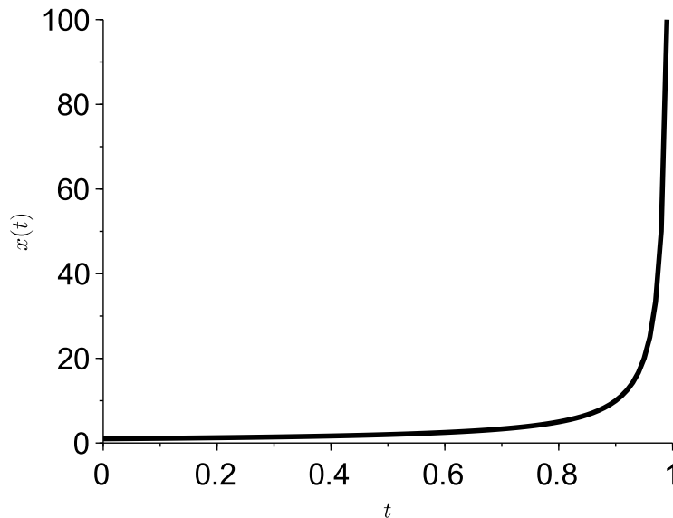
FIGURE 1.1 – On voit dans cette figure le graphe de la solution x(t) du problème de Cauchy (R), la solution est tracée sur [0, z] avec z \approx 1 .
