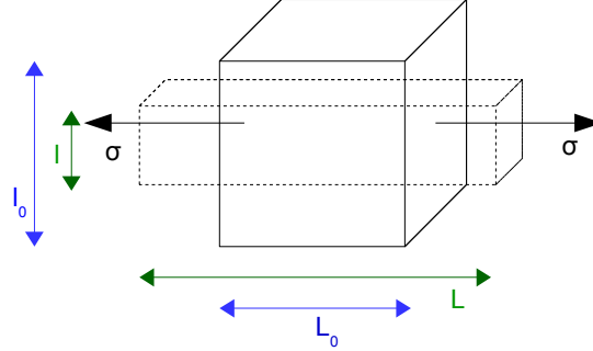
Figure 6 – Element de matière sollicité selon l'axe x par un tenseur de contraintes uniaxial.
