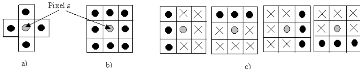
FIGURE 1.10 – Eléments structurants : a) croix 4-connective b) carré 8-connectif c) traits pivotés ( \times =indifférent)
