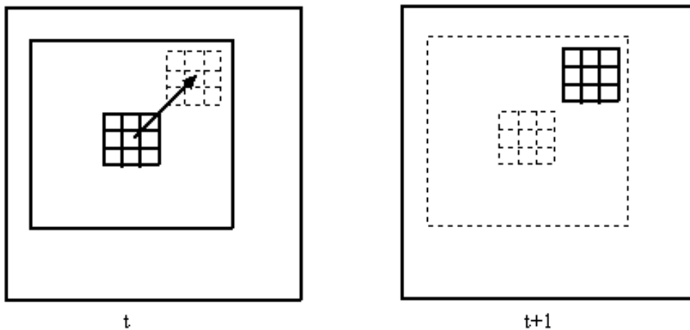
FIGURE 2.20 – Mise en correspondance d'un bloc 3 \times 3
