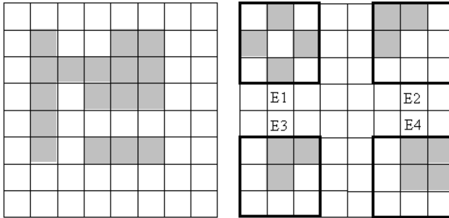
FIGURE 4.37 – a) Forme binaire (en gris) ; b) Eléments structurants.
