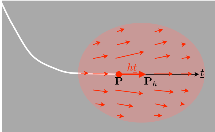
FIGURE 8.4 – Zone de l'objet au voisinage de la pointe de la fissure \mathbf{P} et représentation du champ de vecteur \underline{v} servant à transporter \Omega \setminus \Gamma_h sur \Omega \setminus \Gamma .
