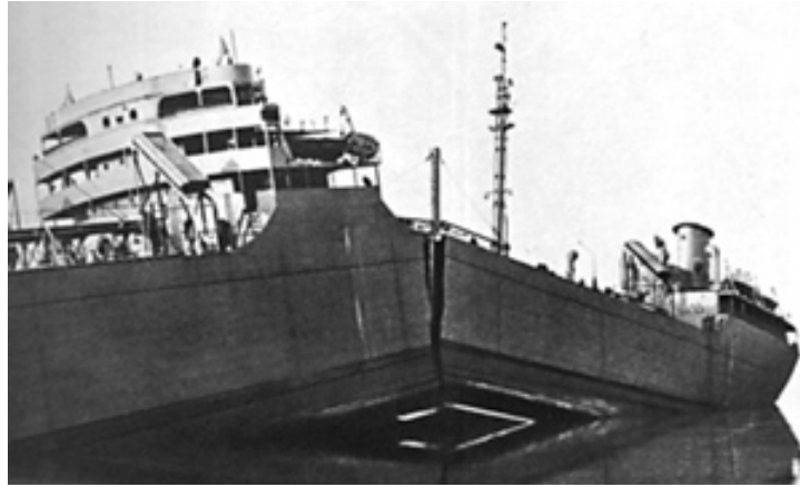
FIGURE 4.9 – Le Schenectady, un des liberty ships entièrement rompus
