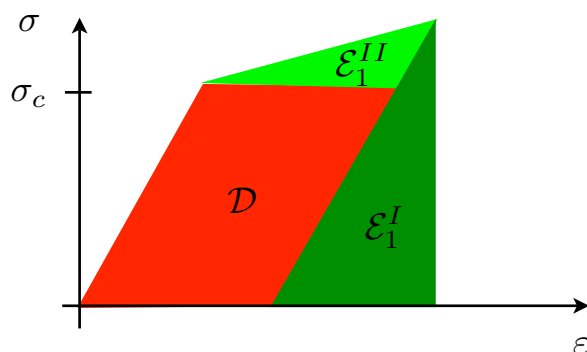
FIGURE 5.10 – Bilan d’ nergie de l’assemblage patin-ressort   la fin de la mont e en charge. En vert fonc  : l’ nergie  lastique stock e dans le premier ressort ; en vert clair : l’ nergie  lastique stock e dans le deuxi me ressort ; en rouge : l’ nergie dissip e par frottement.
